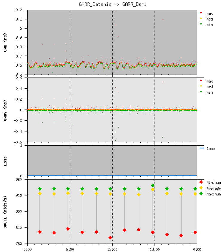
Abbildung 4: Delay und Bandbreitenmessungen
